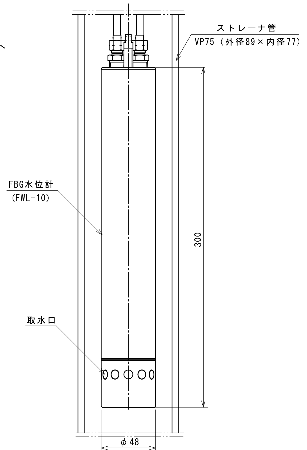
A部詳細：FBG水位計
