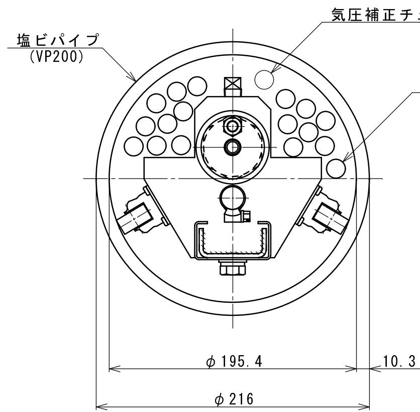
断面図 (1:3)
