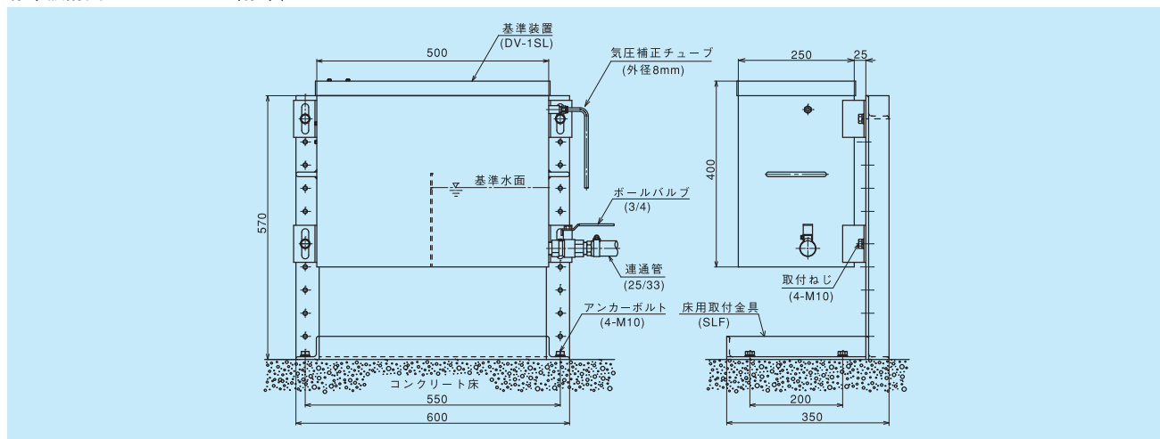
標準設計図 SDV-1SL-B (標準)
