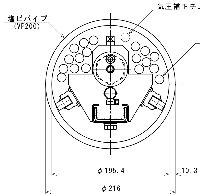
断面図 (1:3)
